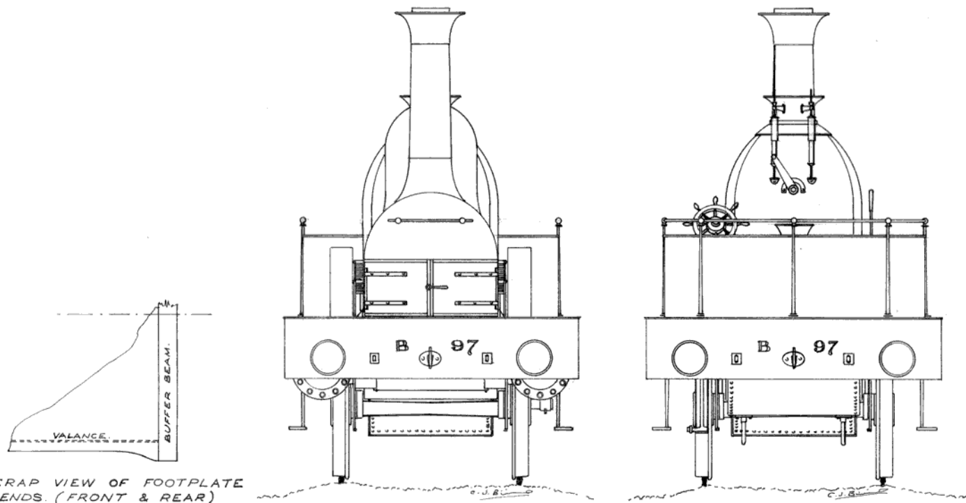
L. B. & S. C. R. 2-2-2T No 97 END VIEWS.
